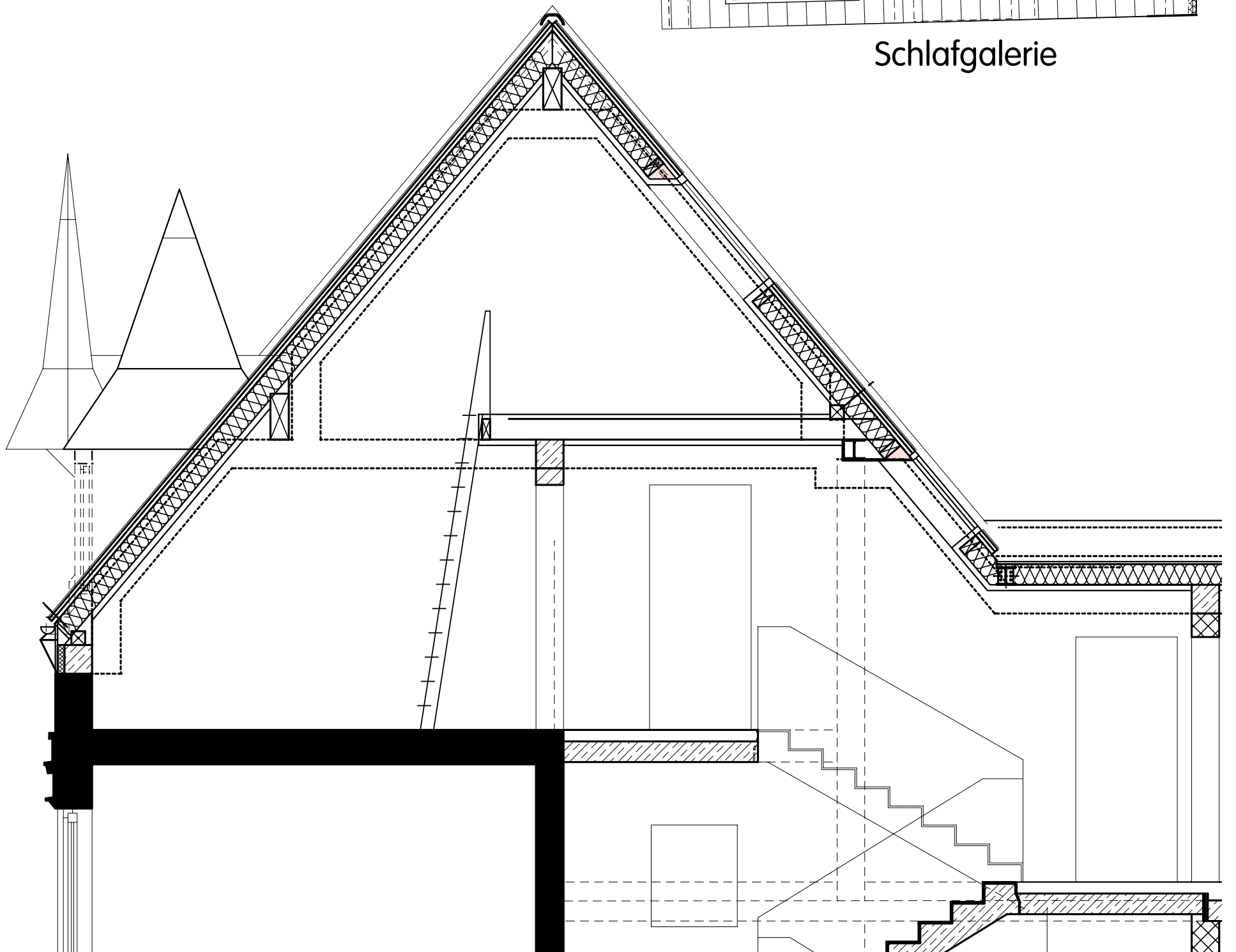
Schnitt
