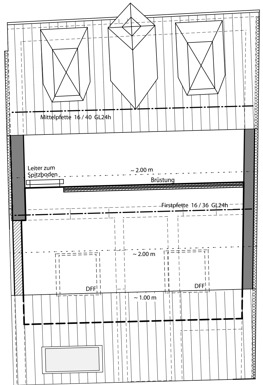
Schlafgalerie
